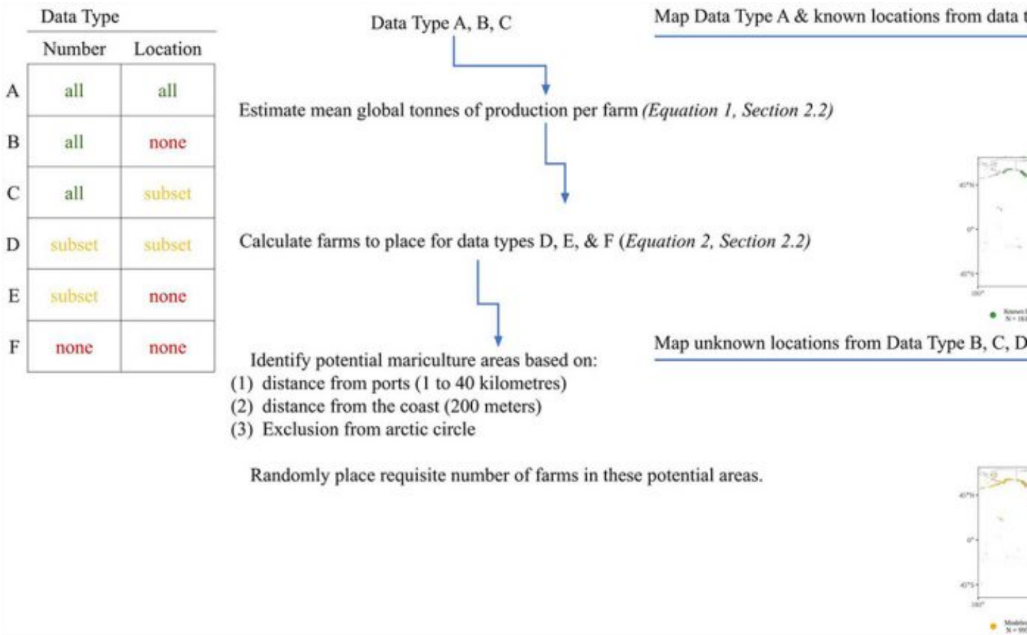
Fig. 1: Esquema del flujo de trabajo necesario para la estimación y el mapeo de cada tipo de datos.
